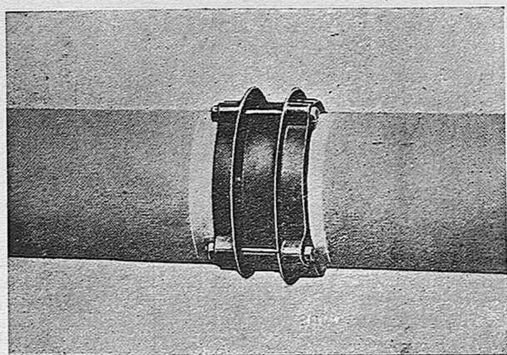
Unión sistema GIBault, montada.
