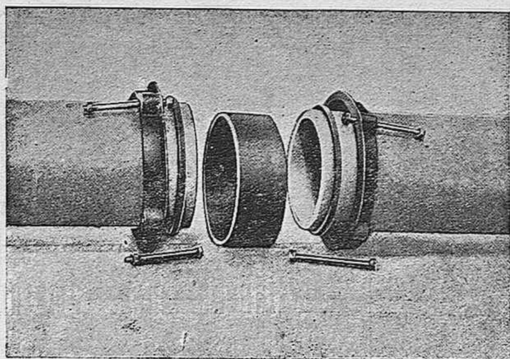
Unión sistema GIBault, desmontada.
