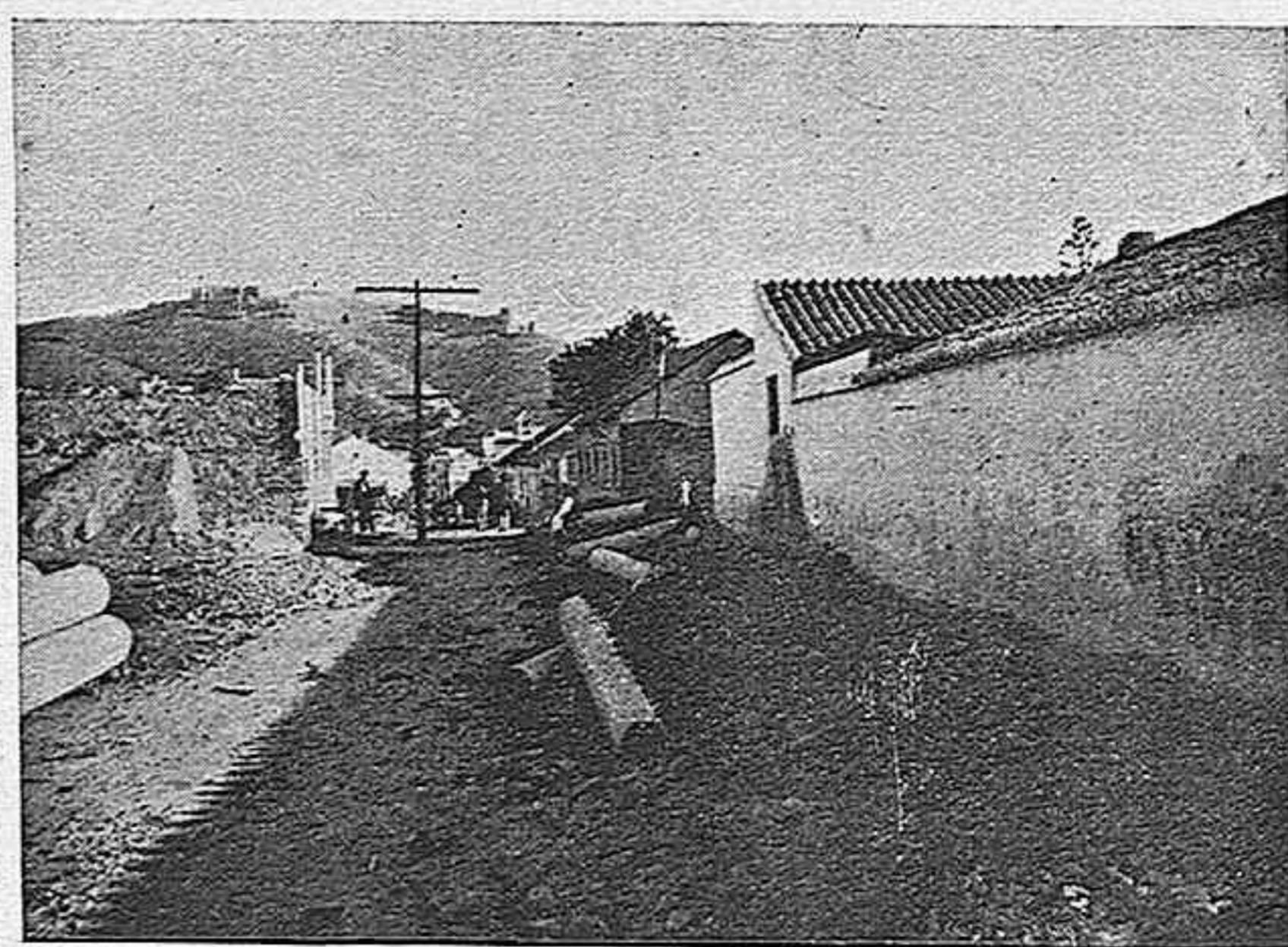
Tubería de 225 m/m instalándose actualmente calle Fernando el Católico, Málaga, para conducción de las aguas potables de Torremolinos.
