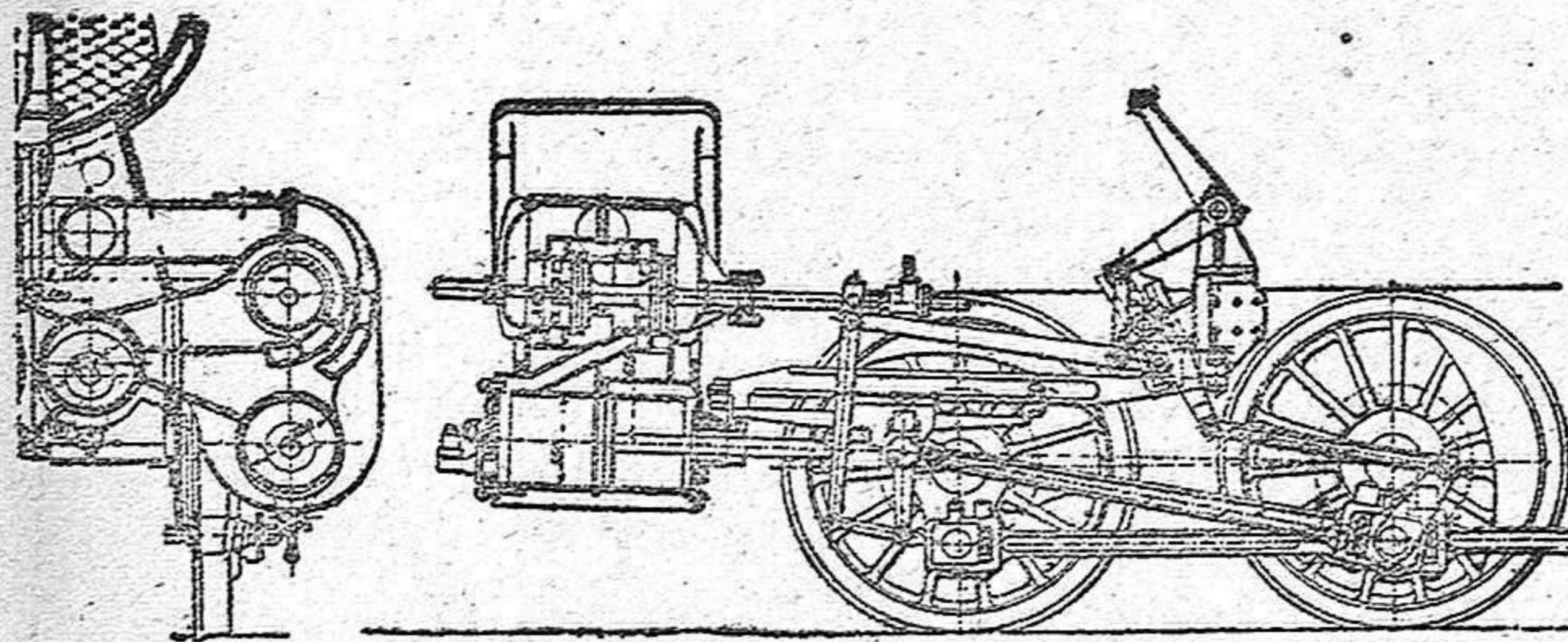
Muestra de grabados.—Disposición del cilindro y del mecanismo de una locomotora COMPOUND.
