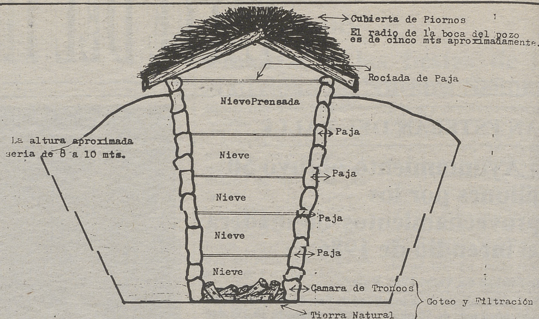
Esquema y funcionamiento de uno de los pozos de Piedralaves: Las primeras cubiertas fueron de piornos, posteriormente se utilizó la teja curva. Cada metro, o metro y medio, depositaban una rociada de paja. Esta, según la dureza de la nieve se colocaba a más o menos altura, entre capa y capa. Durante la dominación árabe el uso de la nieve fue un medio terapéutico habitual. ARCHIVO
