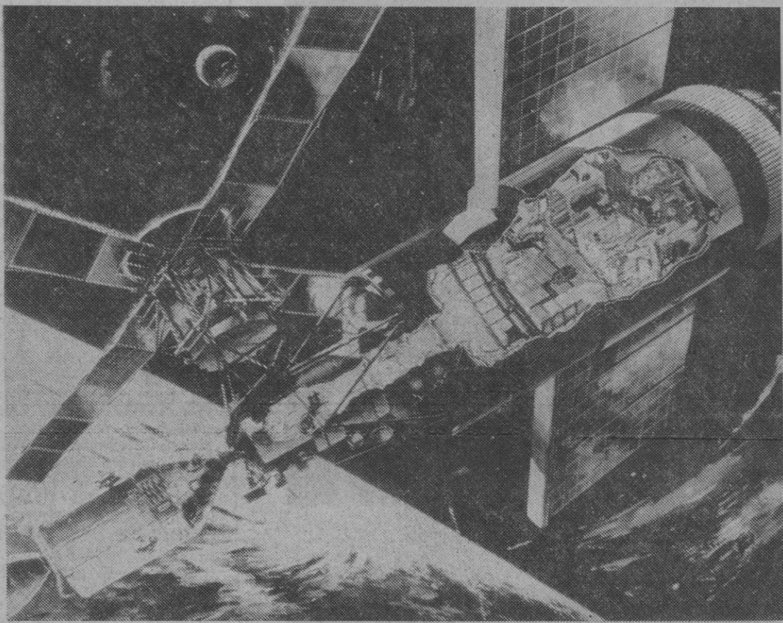
El Skylab aparece en este dibujo totalmente desplegado, ya en órbita terrestre. En la parte inferior izquierda, el módulo de mando-servicio del Apolo. Sobre la nave, el telescopio solar.
