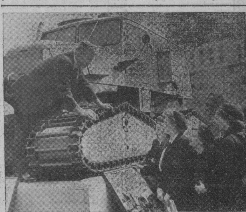
Seis muchachas de escuela escuchan fascinadas las explicaciones del doctor Vivian Fuchs—ahora sir Vivian Fuchs—sobre el funcionamiento del "Haywire", uno de los cuatro vehículos llamados Sno-cats empleados por la Expedición Transantártica, que se han expuesto recientemente en la famosa plaza londinense de Trafalgar. Unos días después de haberse tomado esta fotografía, el "Haywire" inició una gira de cuatro meses por la Gran Bretaña.
