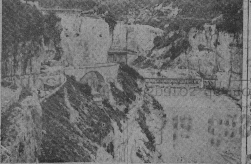
Francia contará en breve con un gigantesco salto de agua, el del portazgo de Genissiat, a través del Rhone, que será el más grande de Europa, después del Dniéper, en Rusia. He aquí una fotografía referente a la construcción de la presa
