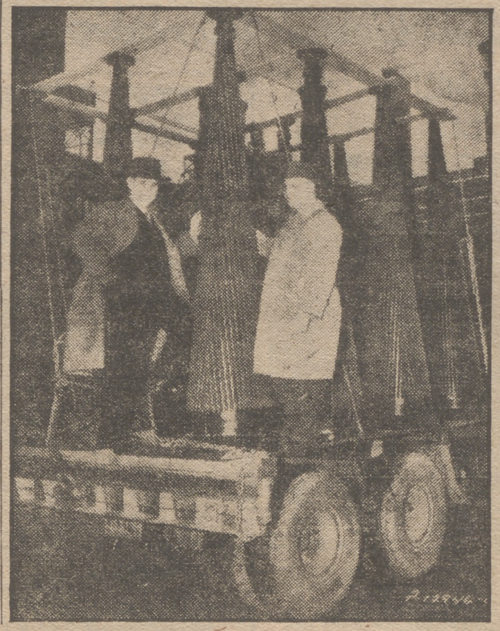
Este artefacto de tan extraño aspecto es un equipo de recogida y purificación de humos y polvo, instalado en el Instituto Edison, del Bronx (Nueva York). Se trata de un prototipo bautizado con el nombre de "Aerodina". El equipo consta de 64 conos de acero, de unos 2,50 metros de altura. Estos conos se instalan a la salida de gases y humos de las calderas. Los vapores entran por la base del cono y salen a través de los 2.000 agujeritos situados en su superficie. El aparato supone una nueva técnica en el servicio de recogida de humos y polvo, y reviste particular importancia en establecimientos como el Edison, a cuyas investigaciones interesa eliminar las materias que pueden perturbarlas. Se debe el nuevo ingenio a un sueco llamado E. T. Linderoth. La máquina cuesta unos 200.000 dólares.
