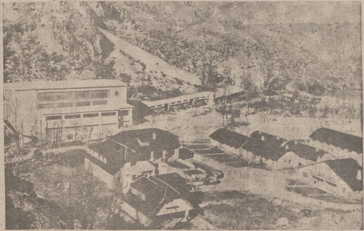
Vista general del poblado y central hidroeléctrica de Moncabril, en Ribadalega, con una potencia de cincuenta y dos mil caballos, capaz de una producción media de 140 millones de kilovatios-hora.
