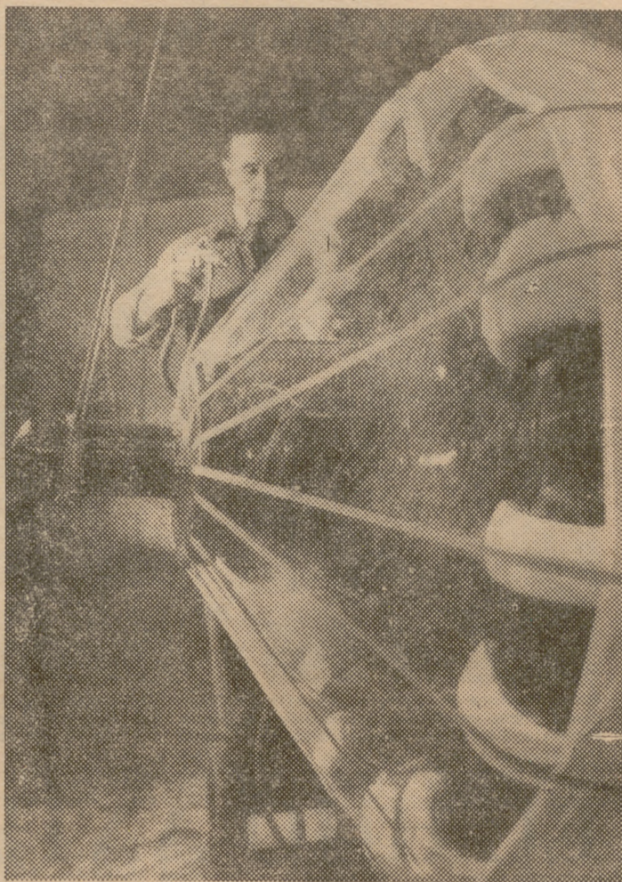
La fotografía ha sido obtenida en los talleres aeronáuticos de la Bristol Aeroplane Com., en Filton (Bristol). Se trata de una complicada operación, a la que son sometidos los motores de aviación para protegerlos contra toda clase de humedad. Esta laboriosa máquina es sólo uno más de los ingenios humanos aplicados a la triunfante industria aeronáutica moderna. (Foto Citra.)
