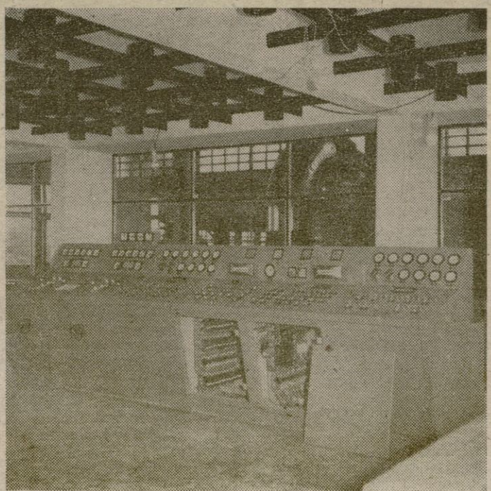
Sala de Mandos Central Eléctrica y Turbinas de Gas de Son Molinas GESA (INI).— Palma.
