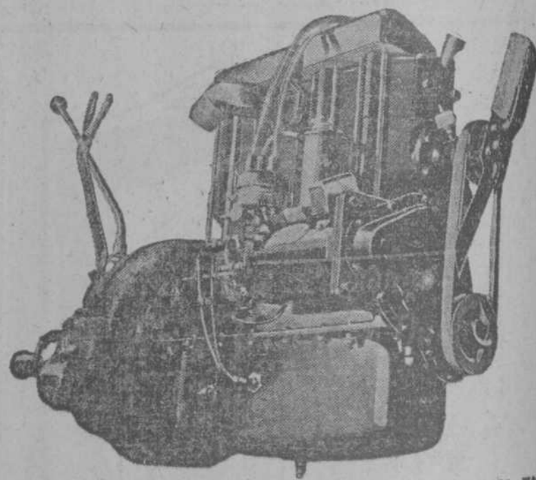
El motor del nuevo tipo Chevrolet ha experimentado notables mejoras mecánicas.
