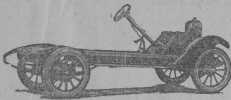
Chasis del nuevo Chevrolet que ha sido notablemente reforzado.
