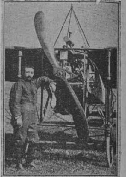
El intrépido aviador leonés D. Enrique Laurín, que se propone hacer el recorrido León-Valadolid-Madrid, habiendo volado ya varias veces con éxito. El Sr. Laurín tripula un magnífico aparato "Blériot" tipo 11, con motor Laboré-Aviation de 46 H-P.
