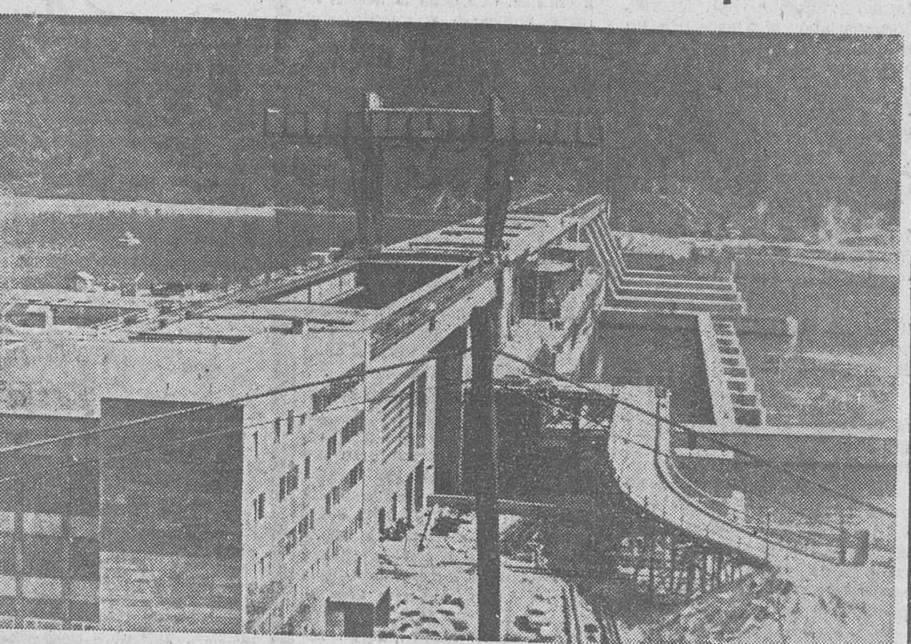
Una vista de la mayor central hidroeléctrica de Europa Central, en el Danubio, junto a Aschach, entre Passau y Linz, que ya está casi terminada. Pertenecer a una compañía austriaca y su capacidad (1.600 millones de kilowatts-hora) es suficiente para abastecer una ciudad como Viena. Las cuatro turbinas, de 75.000 kw. cada una, son movidas por un salto de 16 metros de altura. Las esclusas miden 230 metros de longitud y en la construcción se han empleado 1,2 millones de metros cúbicos de cemento. — (Foto Fiel).
