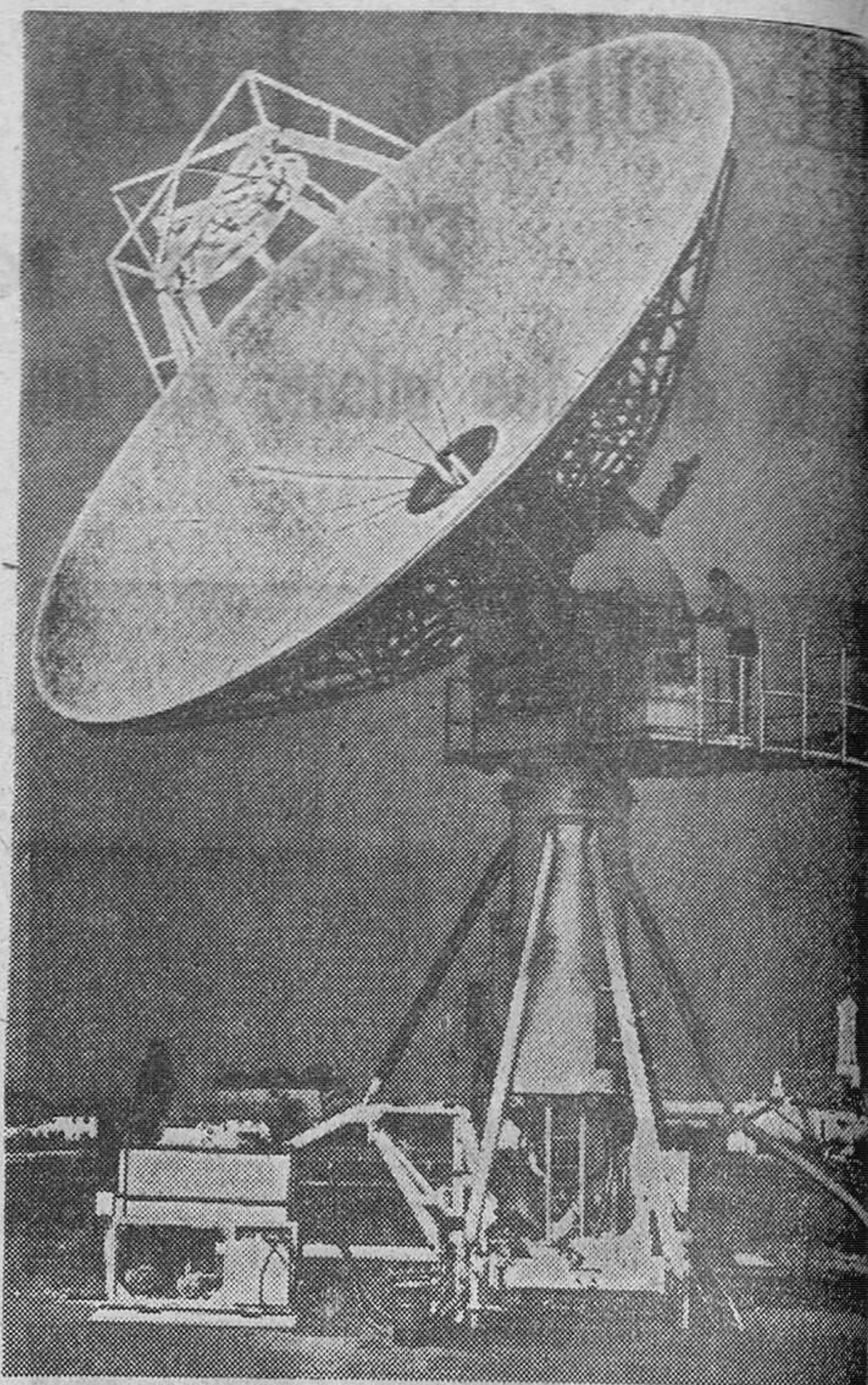
La primera estación terrestre alemana para la transmisión de telefonemas, telexes y datos a través de todos los satélites artificiales del tipo "Telstar" y "Relay" fue inaugurada recientemente. La instalación consiste en una antena de espejos parabólicos de un diámetro de nueve metros y en un remolque para tractores-albarda, en que está instalado el sistema de control y de gobierno.—(Foto DAD)
