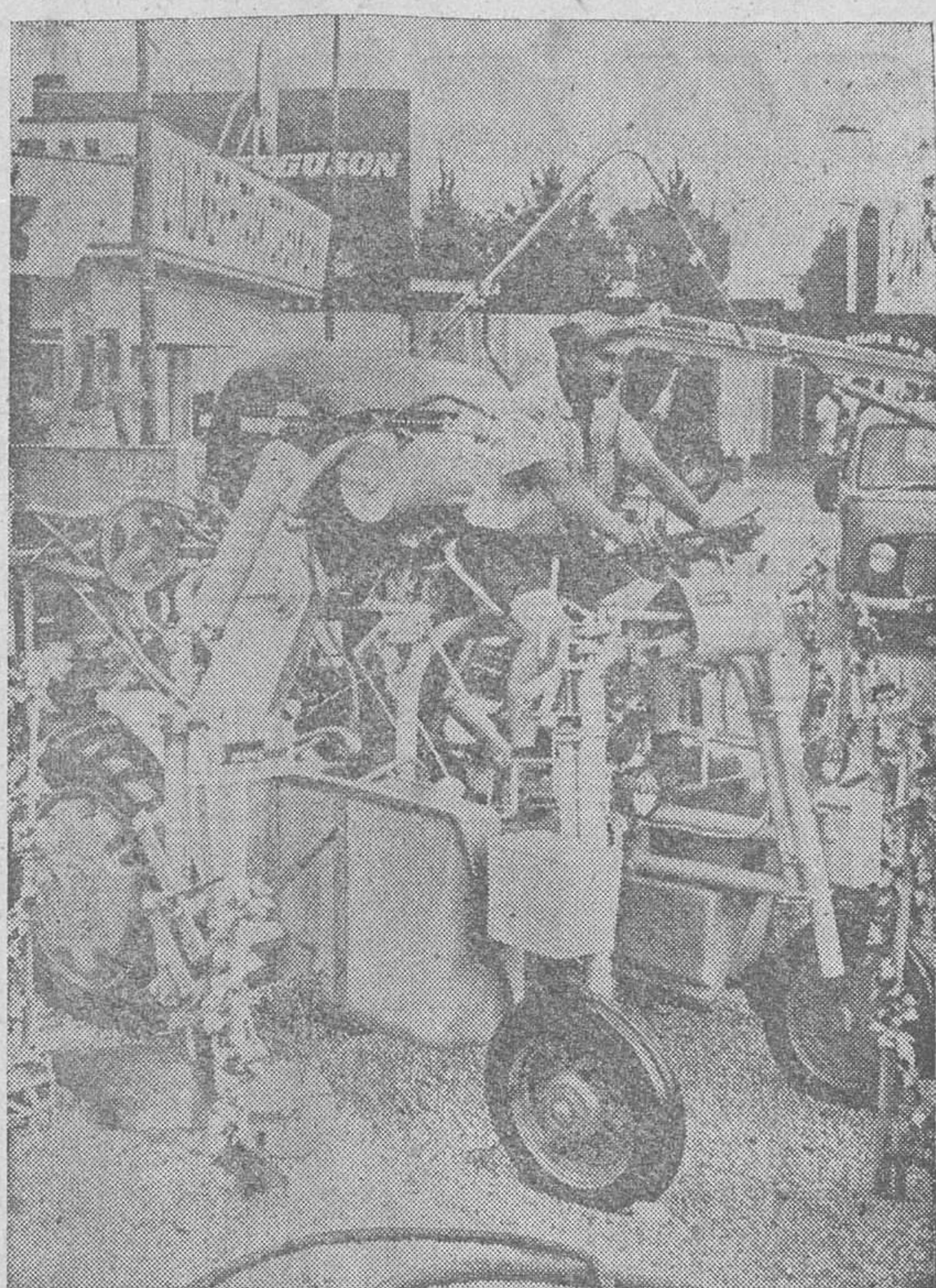
Tractor zancudo En la feria de Otoño de Viena se exhibió por primera vez este tractor de la fotografía. Llamado "tractor zancudo", que permite realizar labores de todo tipo en los viñedos sin dañar las cepas. — (Foto Acala)
