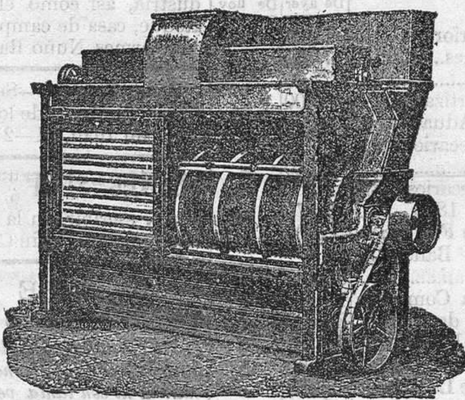
COLUMNA DESPUNTADORA
