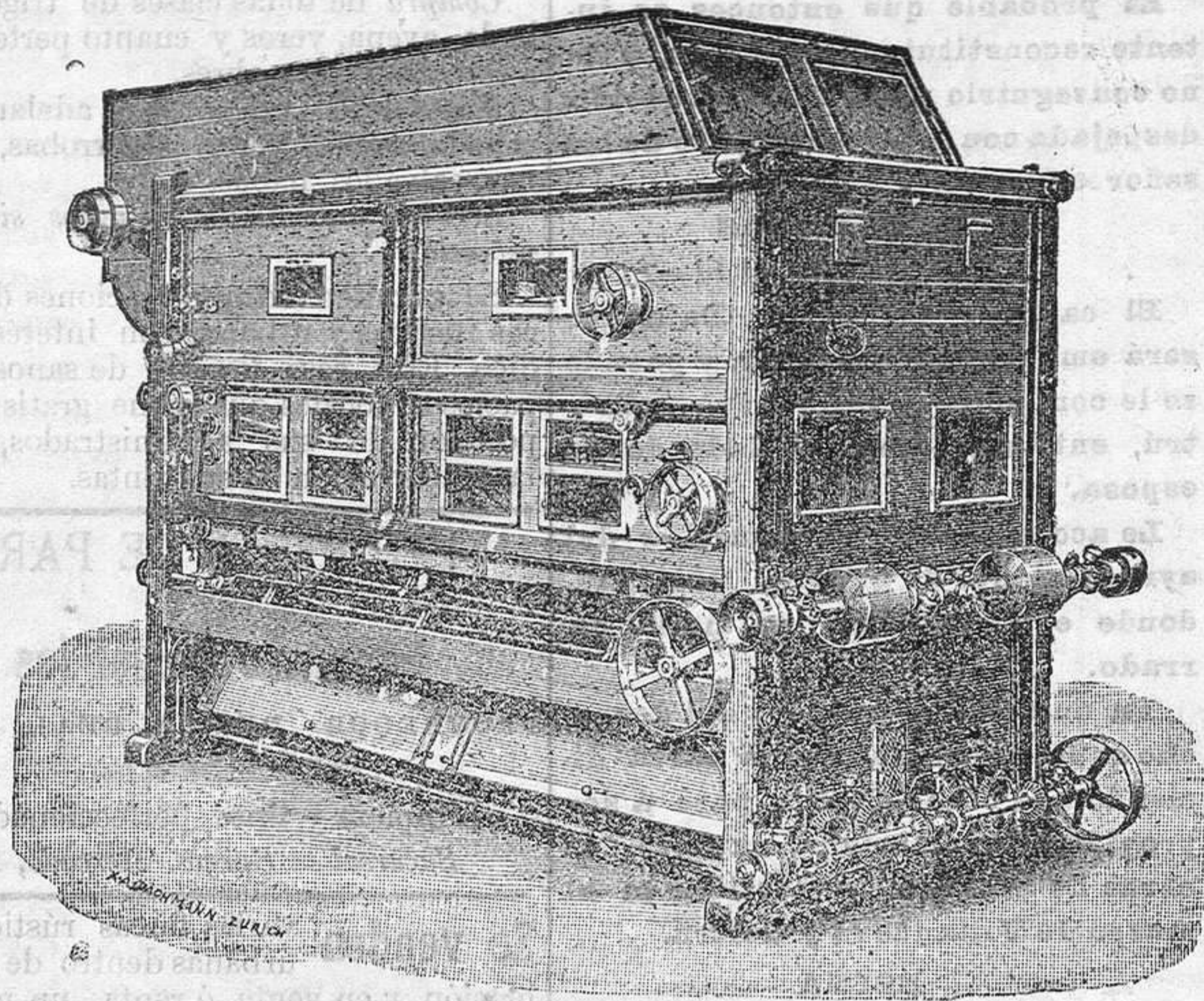
COLUMNA DESPUNTADORA
