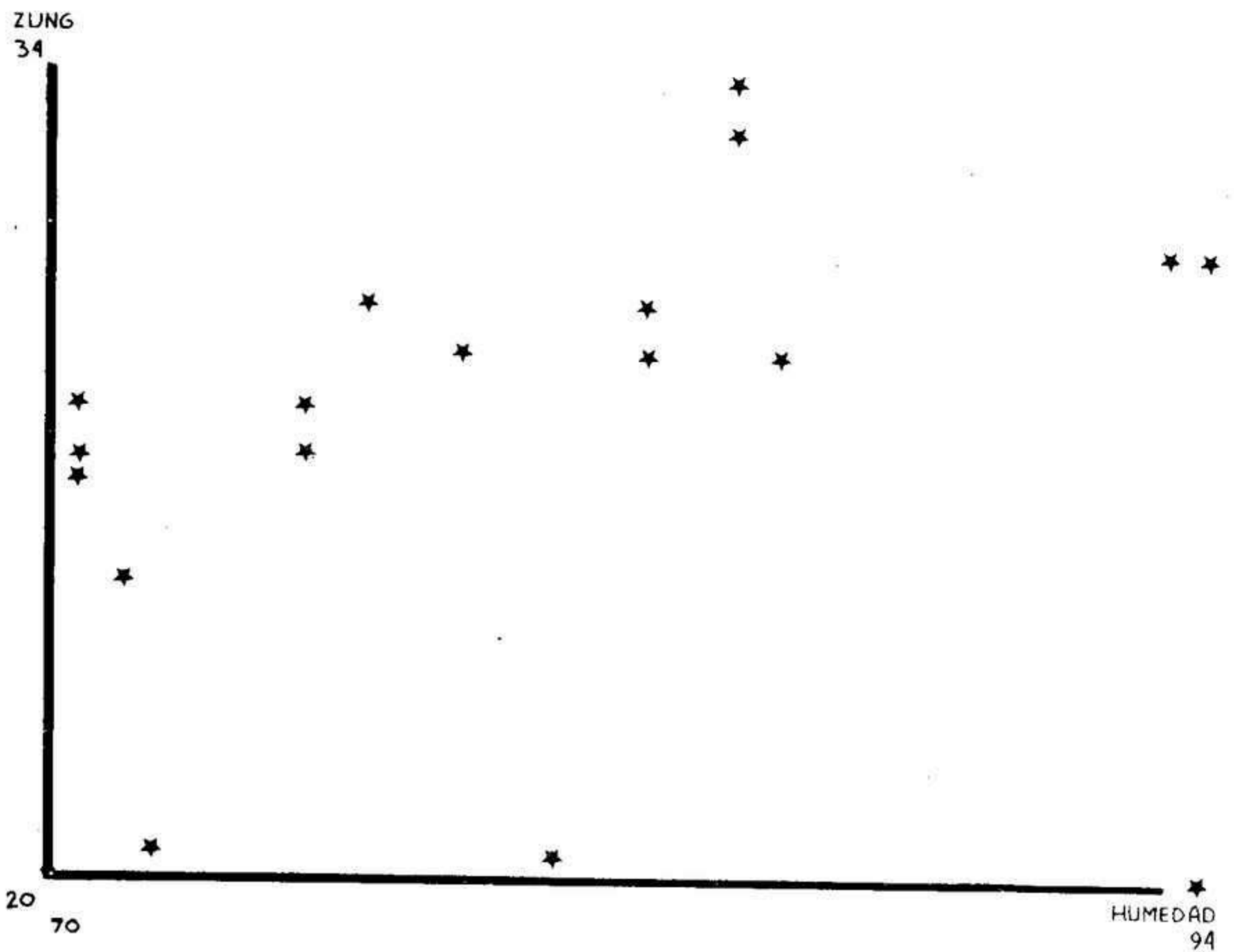
CORRELACION DEPRESION/HUMEDAD RELATIVA EN DICIEMBRE DE 1988
