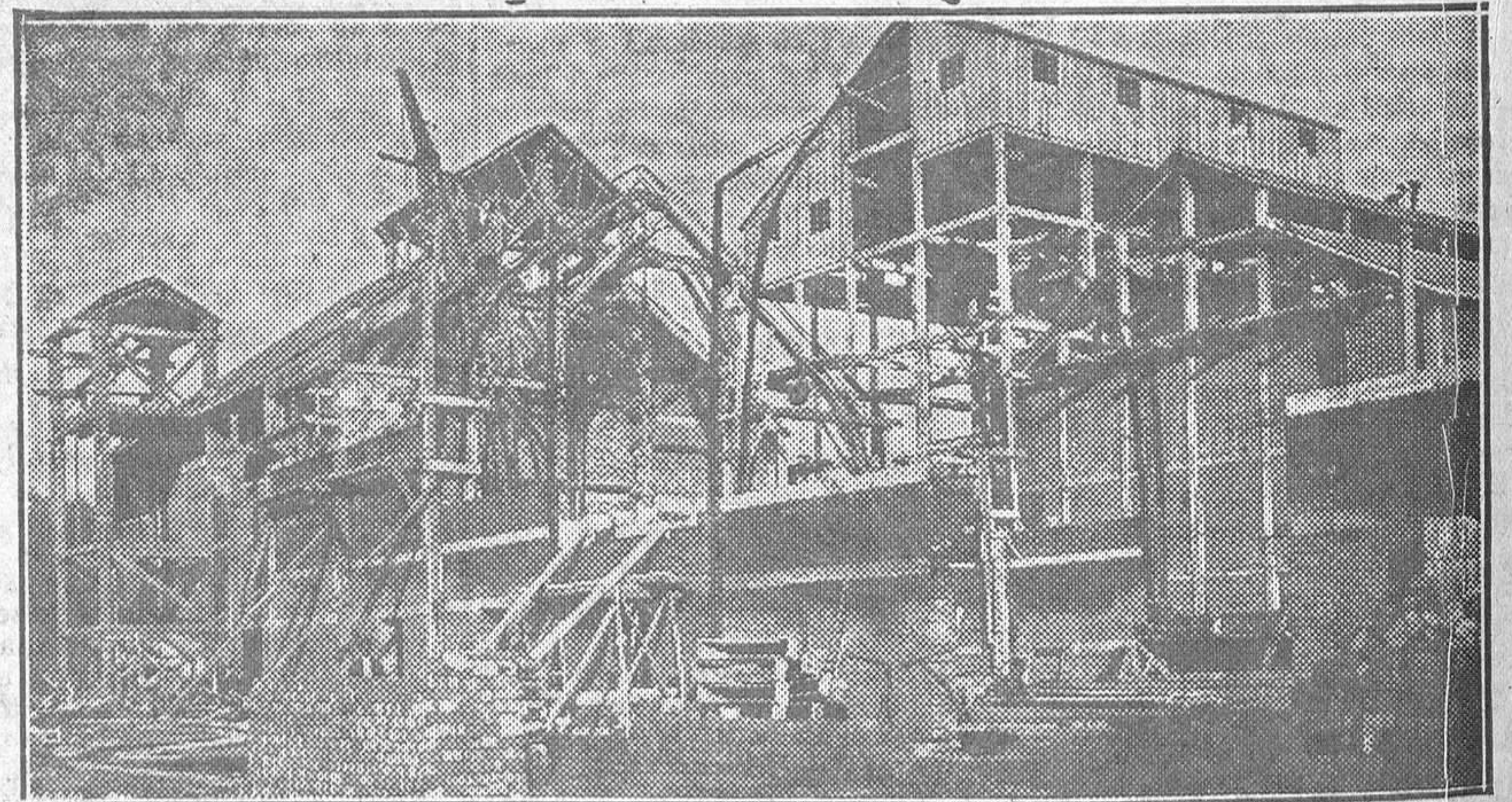
En Octubre de 1924 las obras de la «SOCIEDAD IBERICA DEL NITRÓGENO» llevaban un avance grandísimo
