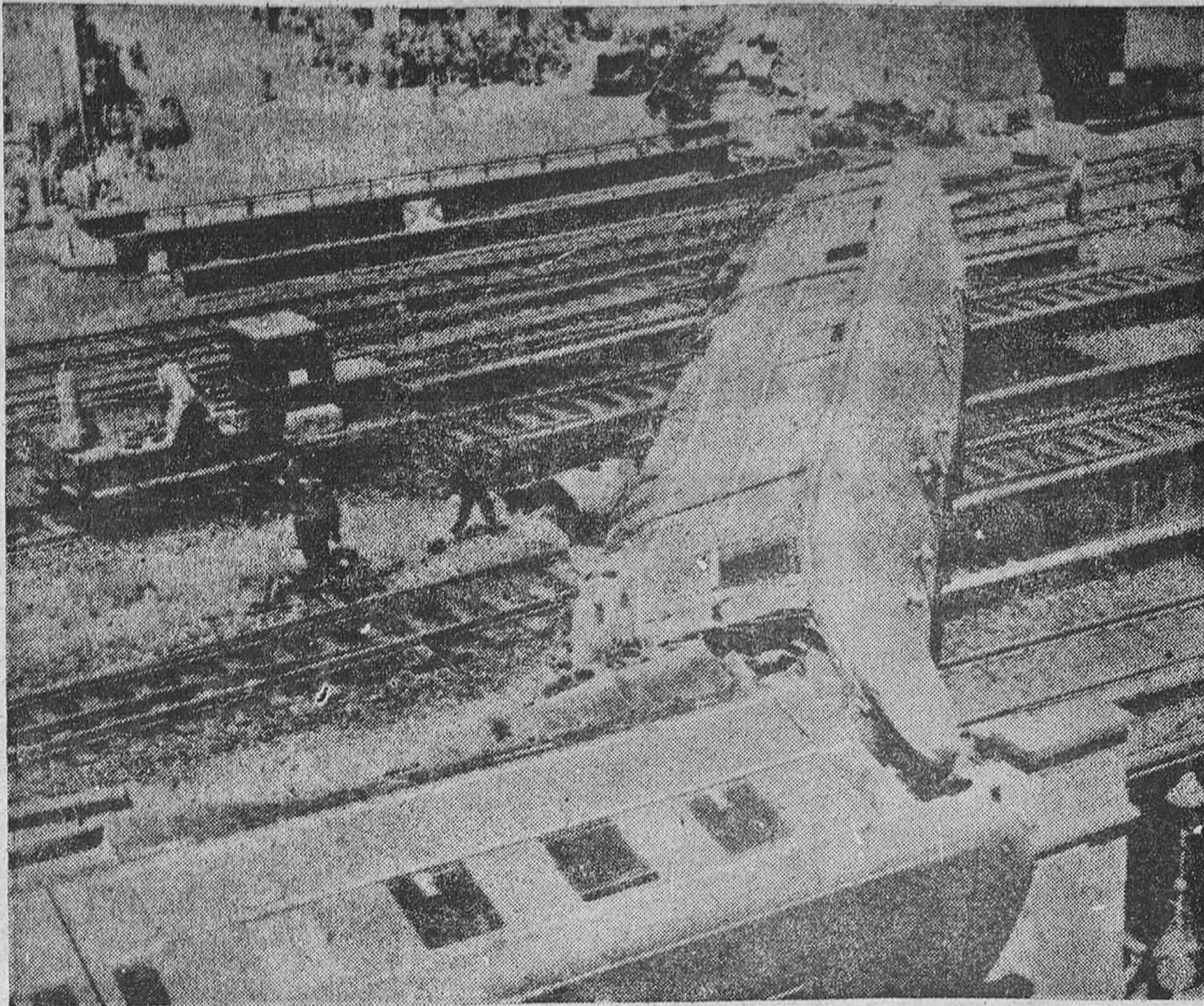
En la estación de Bielefeld (We stfalia), un tren saltó el carril, y como consecuencia hubo que lamentar más de setenta y nueve heridos. El convoy quedó volcado sobre un puente.
