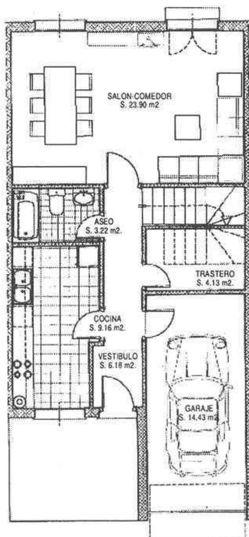
PLANTA BAJA
