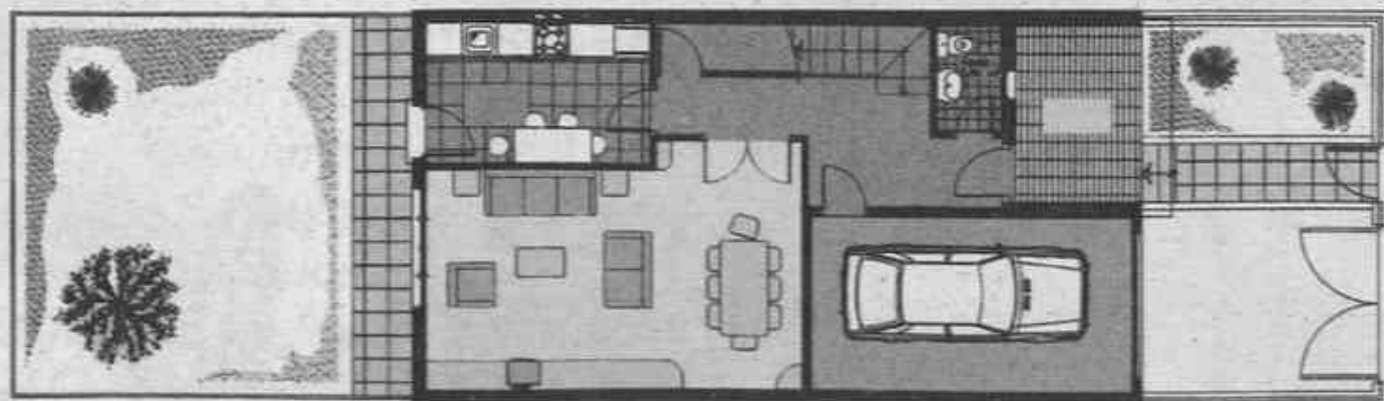
Planta BAJA
