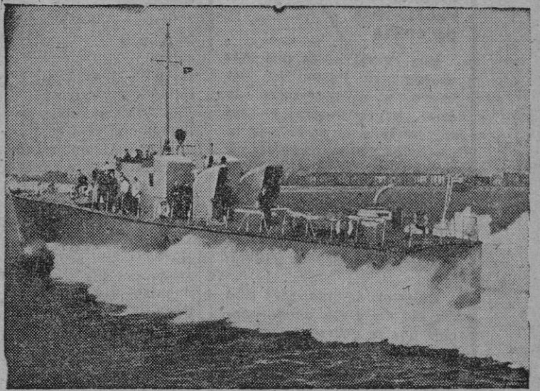
El "Celerity" primer barco de la Armada inglesa propulsado por motores de aviación refrigerados por aire. Tiene un radio de acción de 4.200 millas y la foto nos lo muestra en una carrera de pruebas. -- (Galpe)
