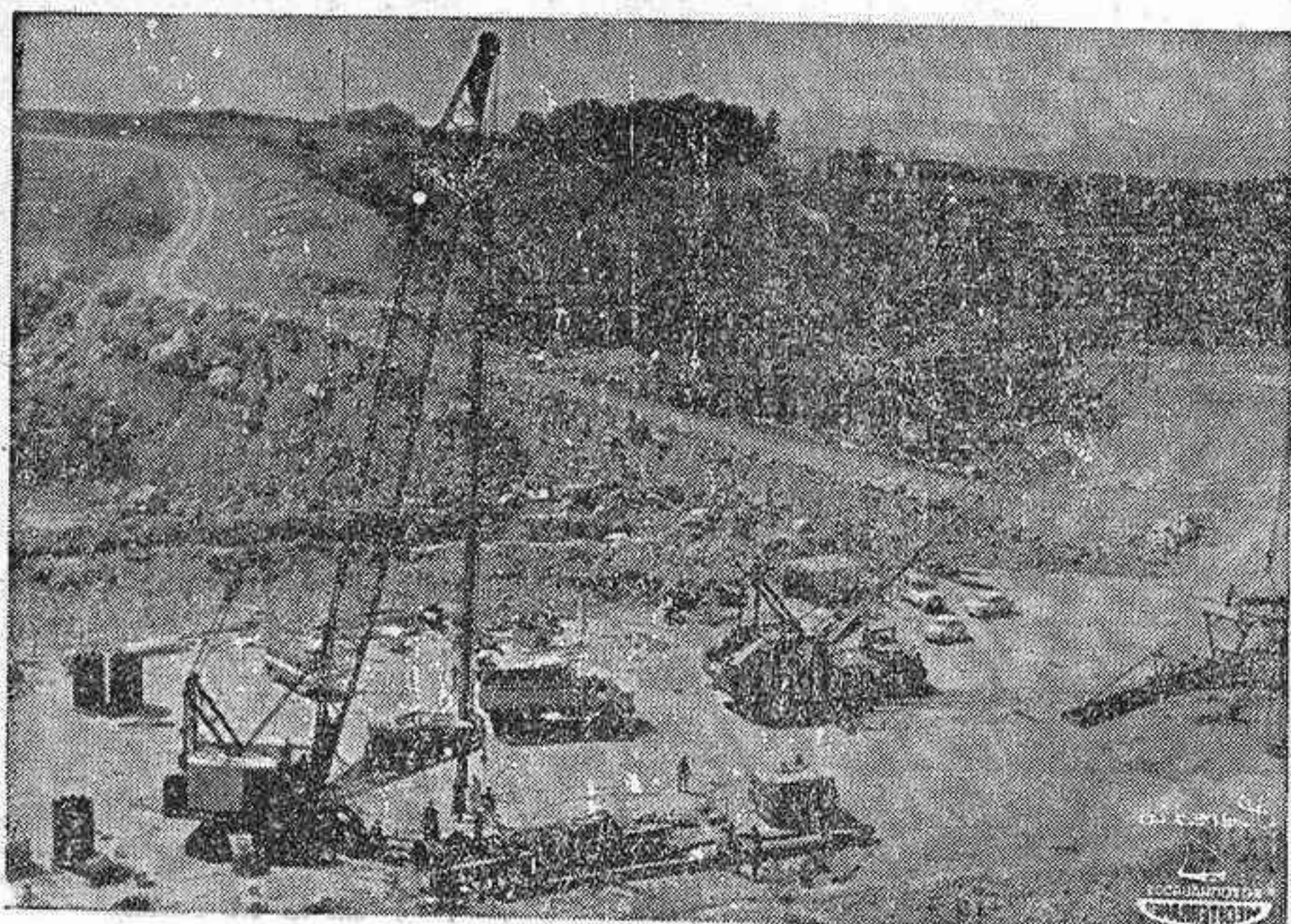
Las obras de la autopista Tarragona-Valencia siguen su marcha a todo ritmo. En la fotografía, los trabajos iniciales, con grúas de enormes dimensiones, para la construcción del gran puente sobre el río Mijares en las inmediaciones del complejo de la Virgen de Gracia, unos cuatrocientos metros río arriba
