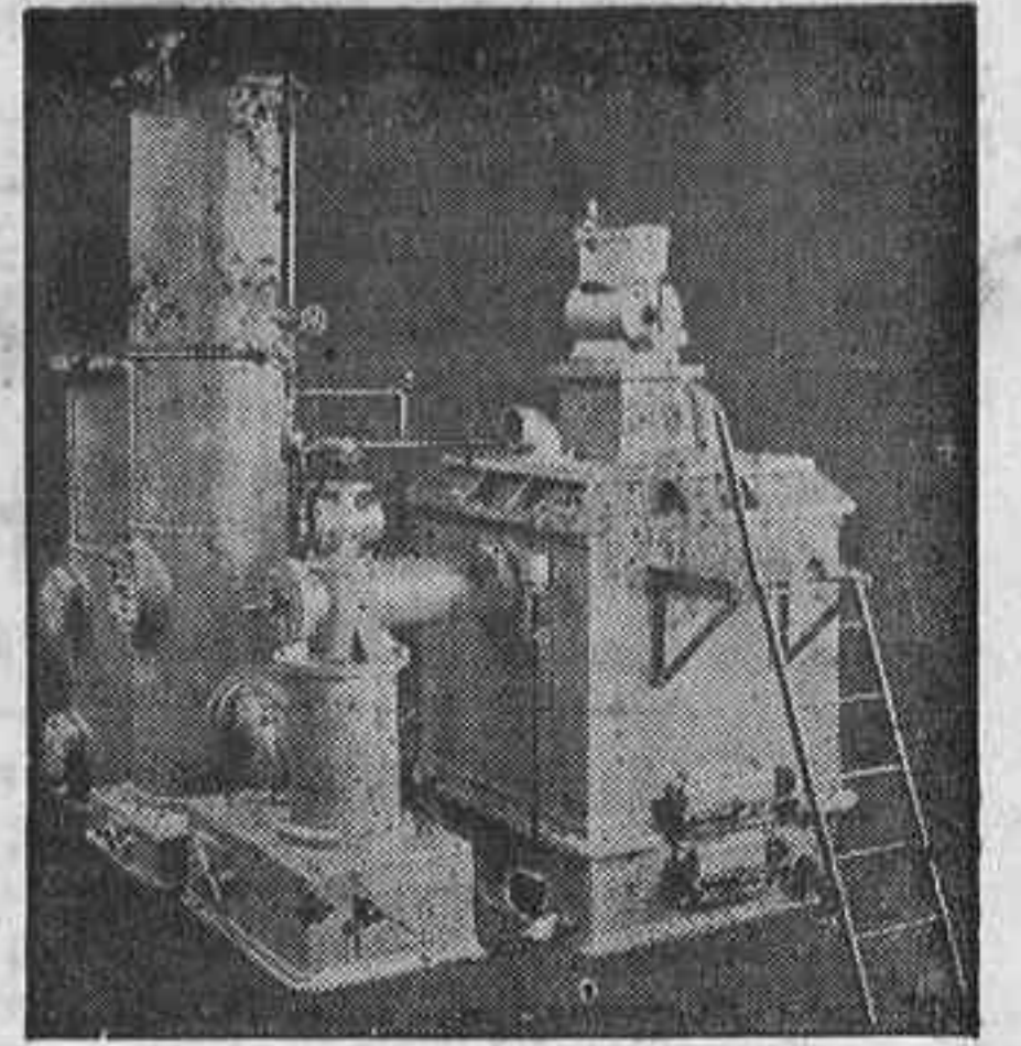
Gasógeno sencillo
