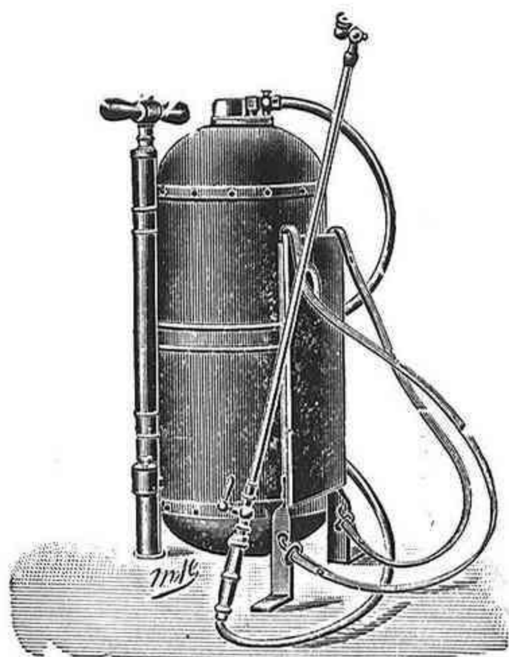
Sulfatadora MURATORI
