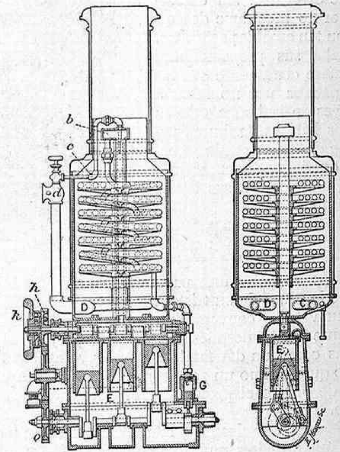
Figs. 2 y 3. Secciones de la caldera y de la máquina del vapor de aluminio
