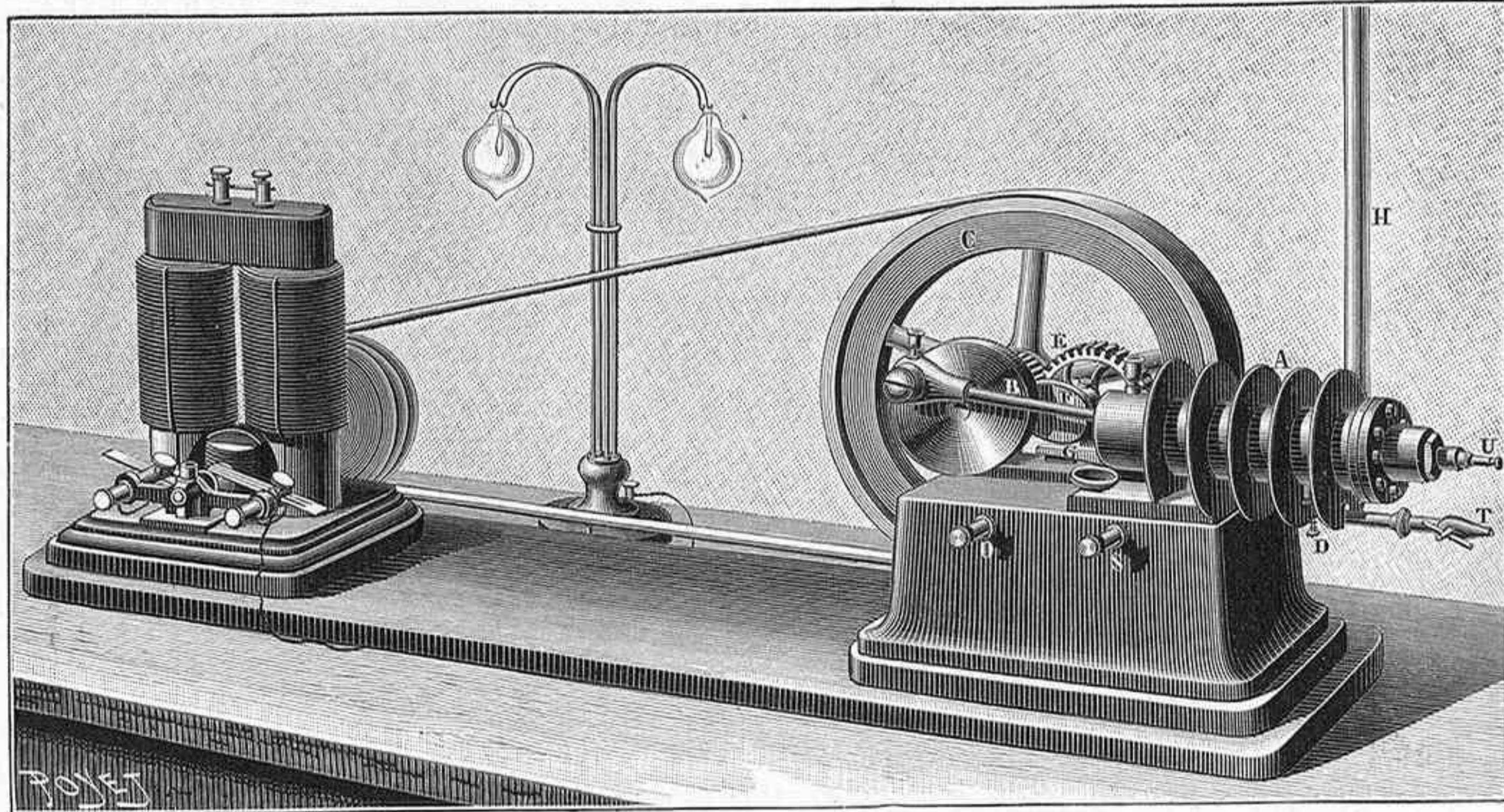
Pequeño motor de gas de una potencia de 5 kilográmetros por segundo, unido á una dinamo
