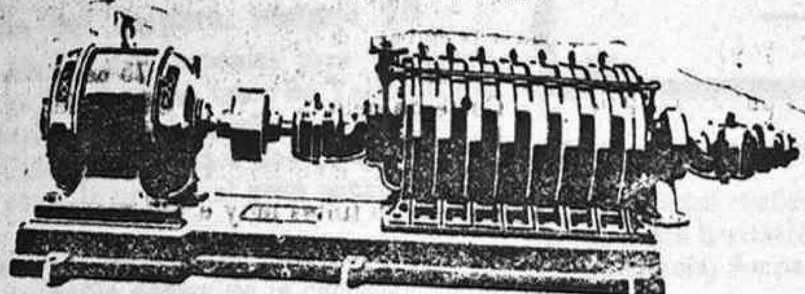
Grupo electro bomba de alta presión
