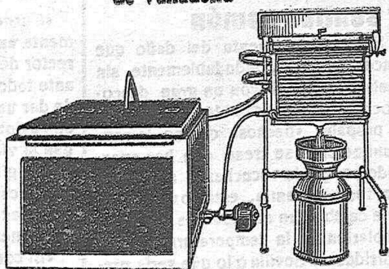
Instalación enfriadora y conservadora de leche
