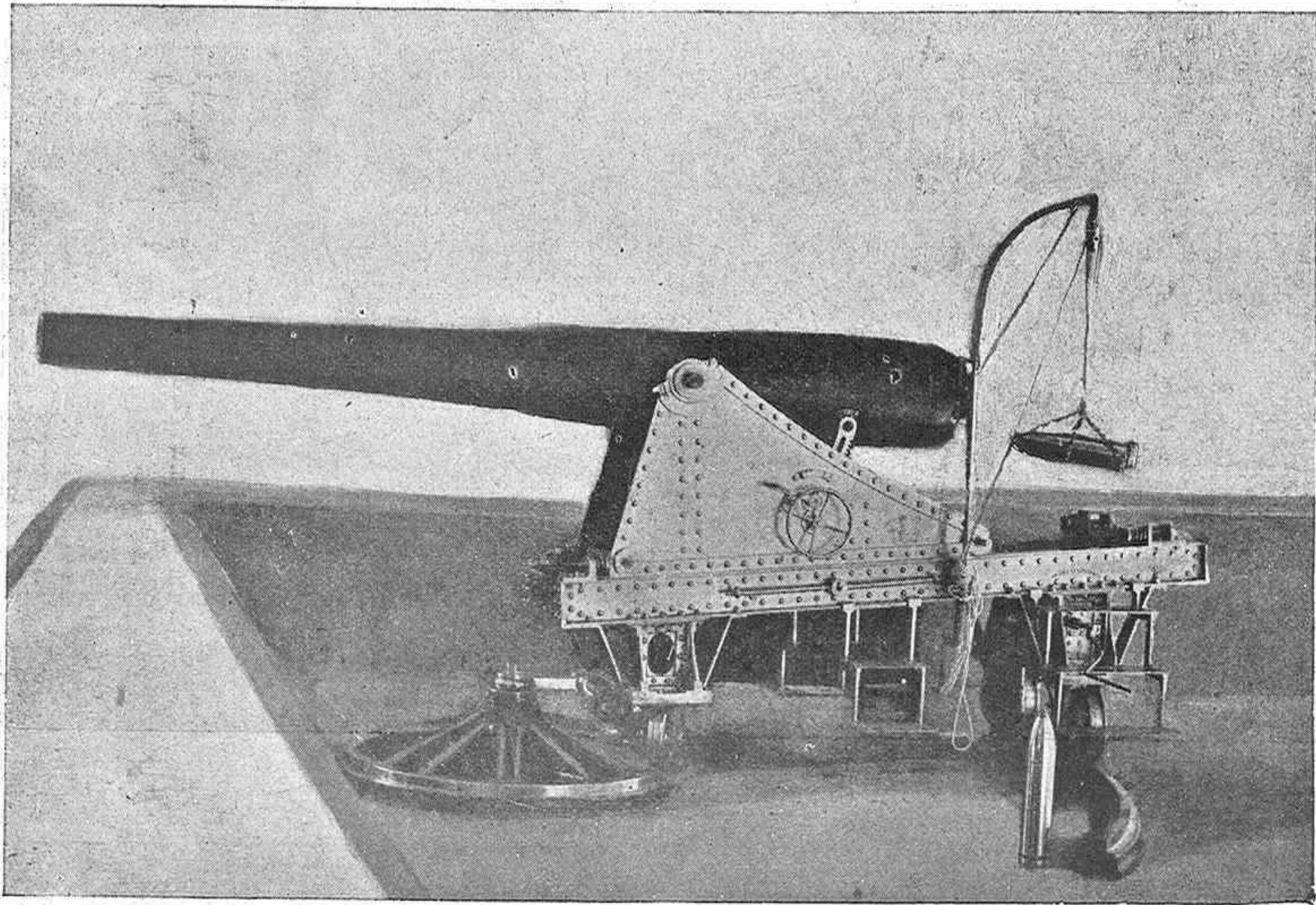
CAÑÓN ORDÓÑEZ, DE 15 CENTÍMETROS
