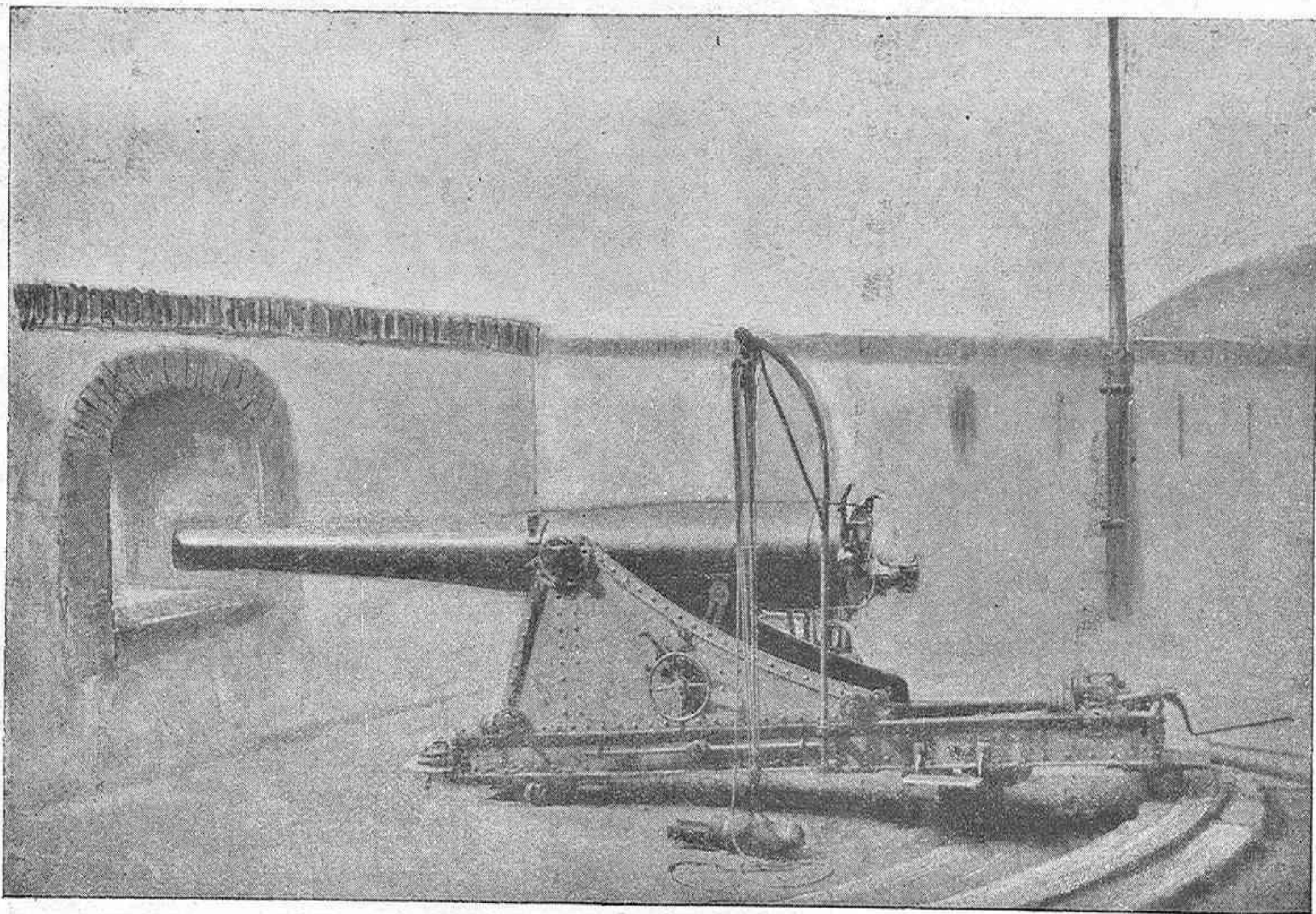
CAÑÓN ORDÓÑEZ, DE HIERRO ENTUBADO, DE 15 CENTÍMETROS, PARA CASAMATA
