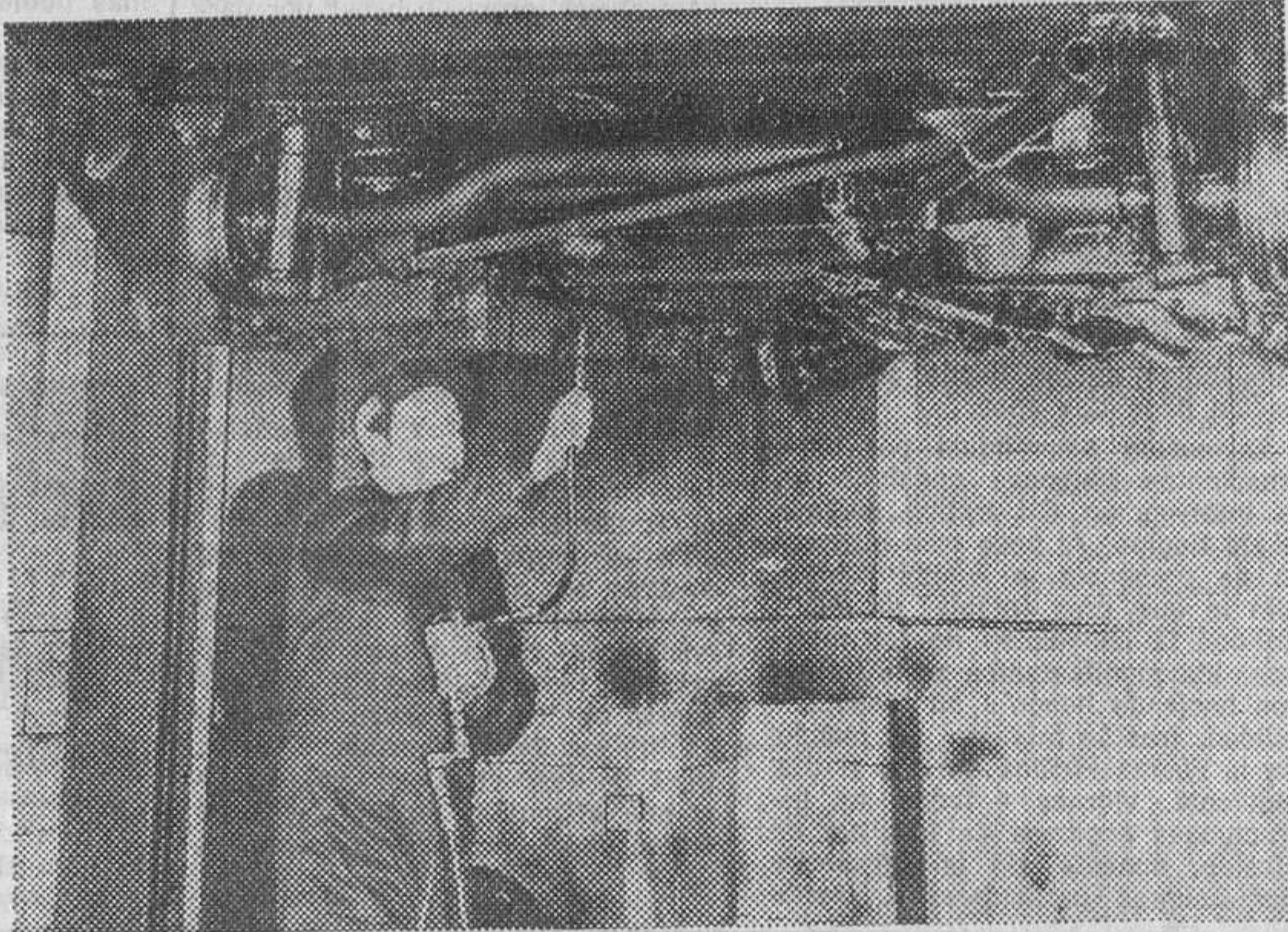
Inyección Dinitrol ML en el faldón del chasis
