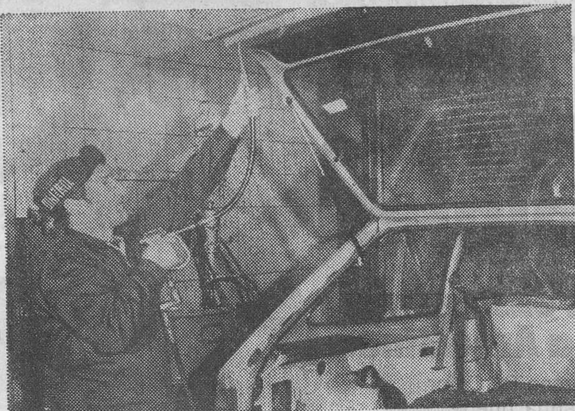
Inyección Dinitrol ML en la tapa portamaletas
