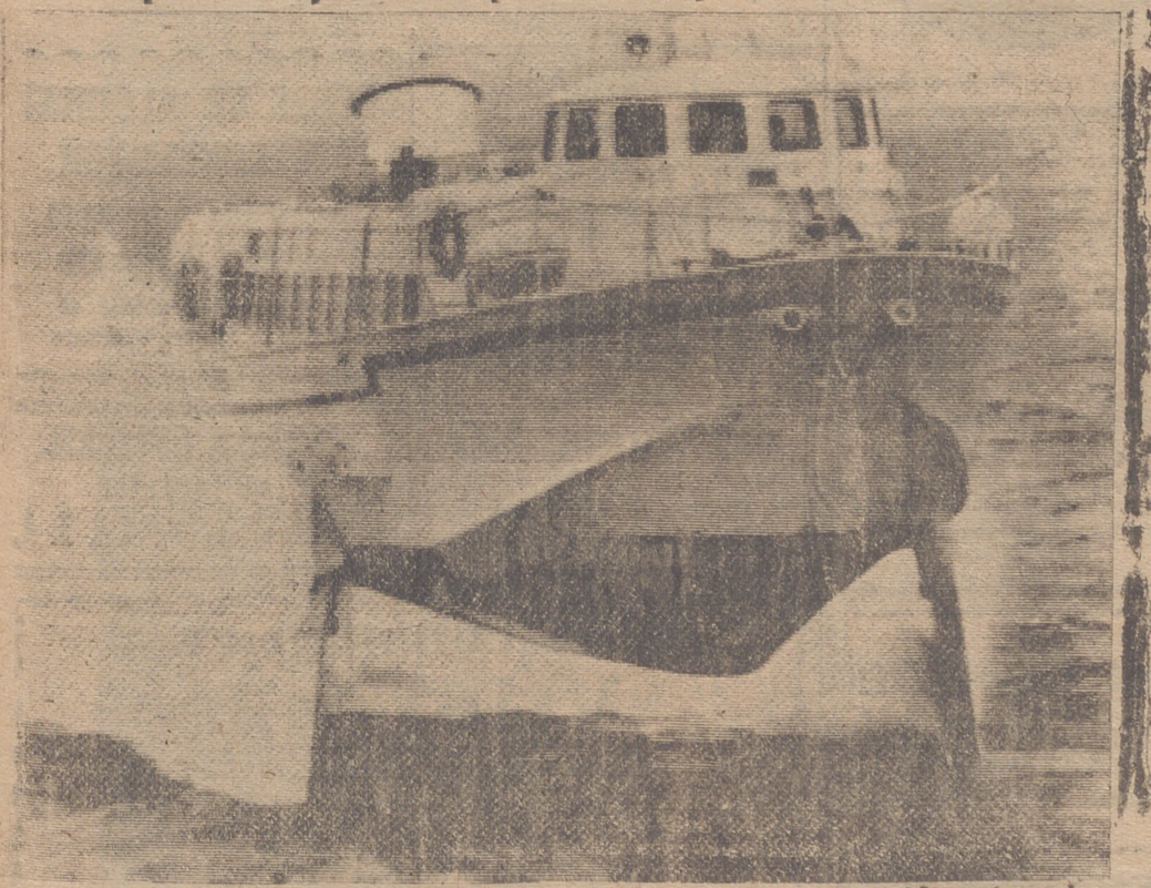
Este es el buque hidroala "Corsario Negro" que ha sido entregado a sus armadores, la empresa naviera española "Marítima Amatares, S. A.", que proyecta dedicarlo al tráfico de pasajeros en las Islas Canarias. Este buque ha sido construido en Hamburgo con patente USA por los astilleros Blohm and Voss y fue bautizado con el citado nombre, siendo madrina la señora marquesa de Taurisano. La fotografía está obtenida con ocasión de las pruebas de mar. Se le considera como el primer buque hidroala apto para la navegación de alta mar. (Foto "Cifra")
